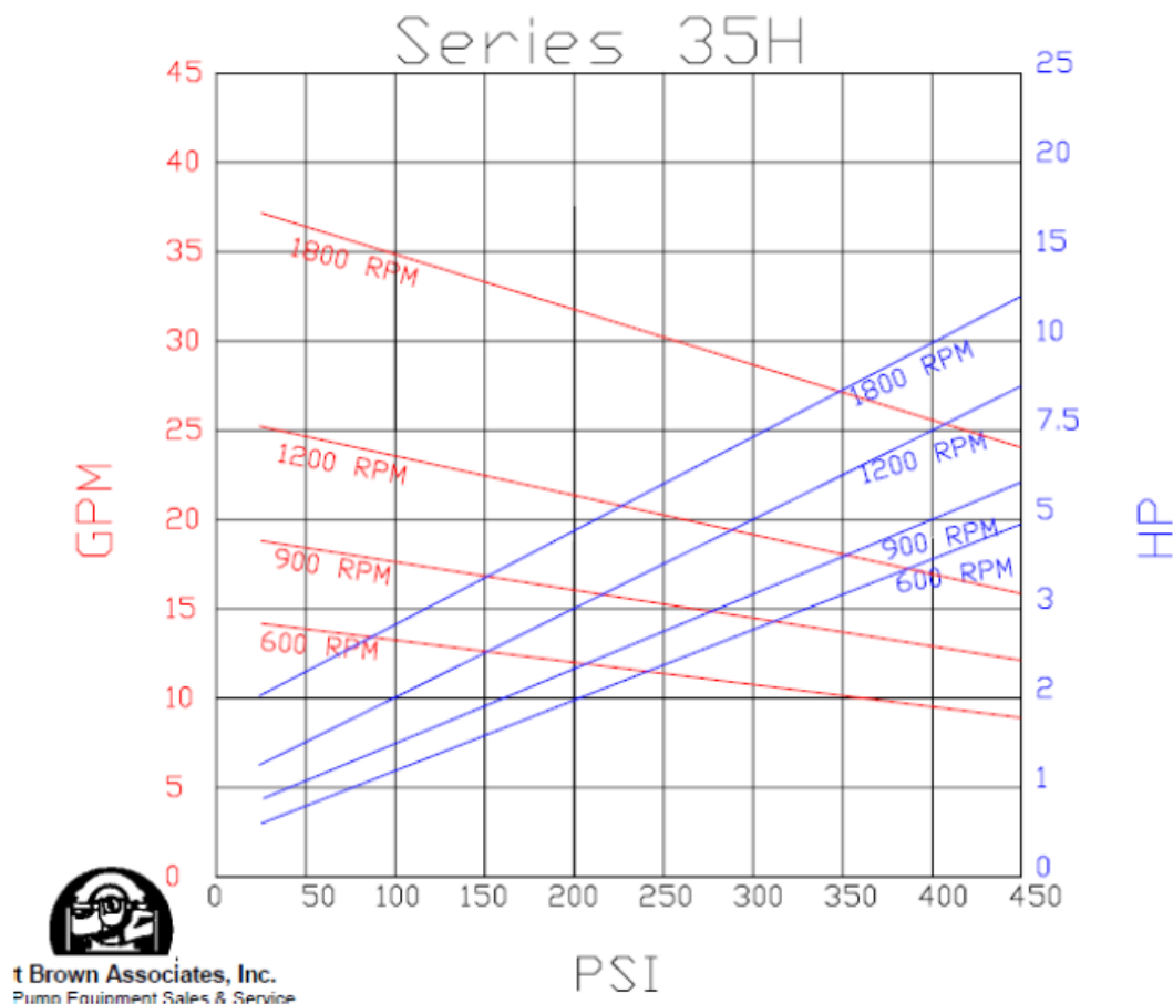
Curva bomba Albany serie H 35
